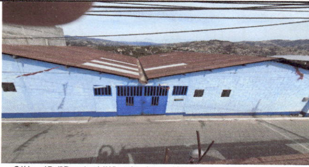
C:\Users\Delin\Downloads\WhatsApp Image 2025-03-25 at 6.17.24 PM (1).jpeg Foto1: Sustritióñ de làmina, por làmina troquelada aluzinc calibre 26
